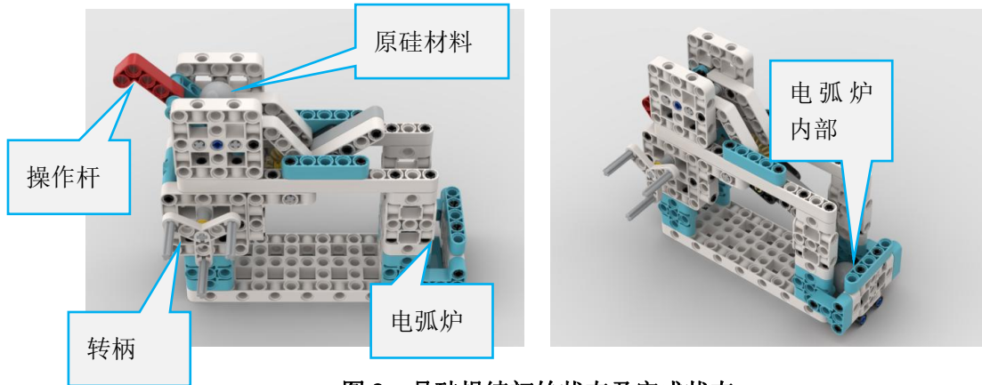
图 8：晶硅提纯初始状态及完成状态
